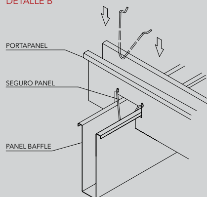
DETALLE B
