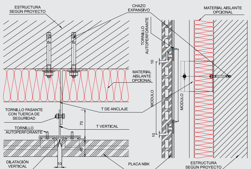
SECCIÓN HORIZONTAL POR FIJACIÓN
