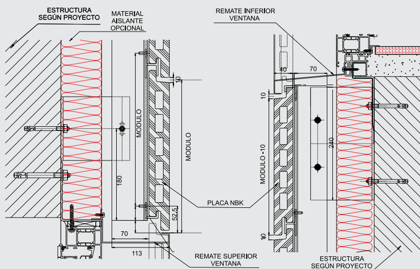
REMATE SUPERIOR DE VENTANA
