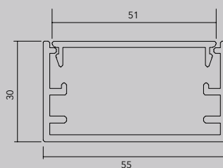
PERFIL HEAVY DUTY (VERTICAL) Material: Aluminio Terminación: Anodizado o pintado Largo máximo 5000mm
