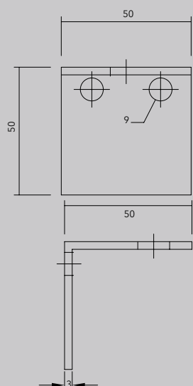
PERFIL ESCUADRA
