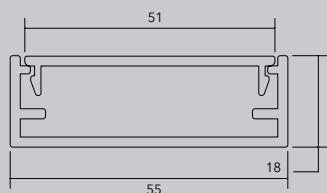
PERFIL SLIMLINE (VERTICAL) Material: Aluminio Terminación: Anodizado o pintado Largo máximo 4000mm
