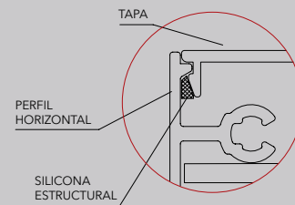
DETALLE C
