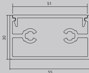
PERFIL HORIZONTAL Material: Aluminio Terminación: Anodizado o pintado Largo máximo 3000mm
