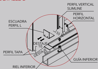
DETALLE B
